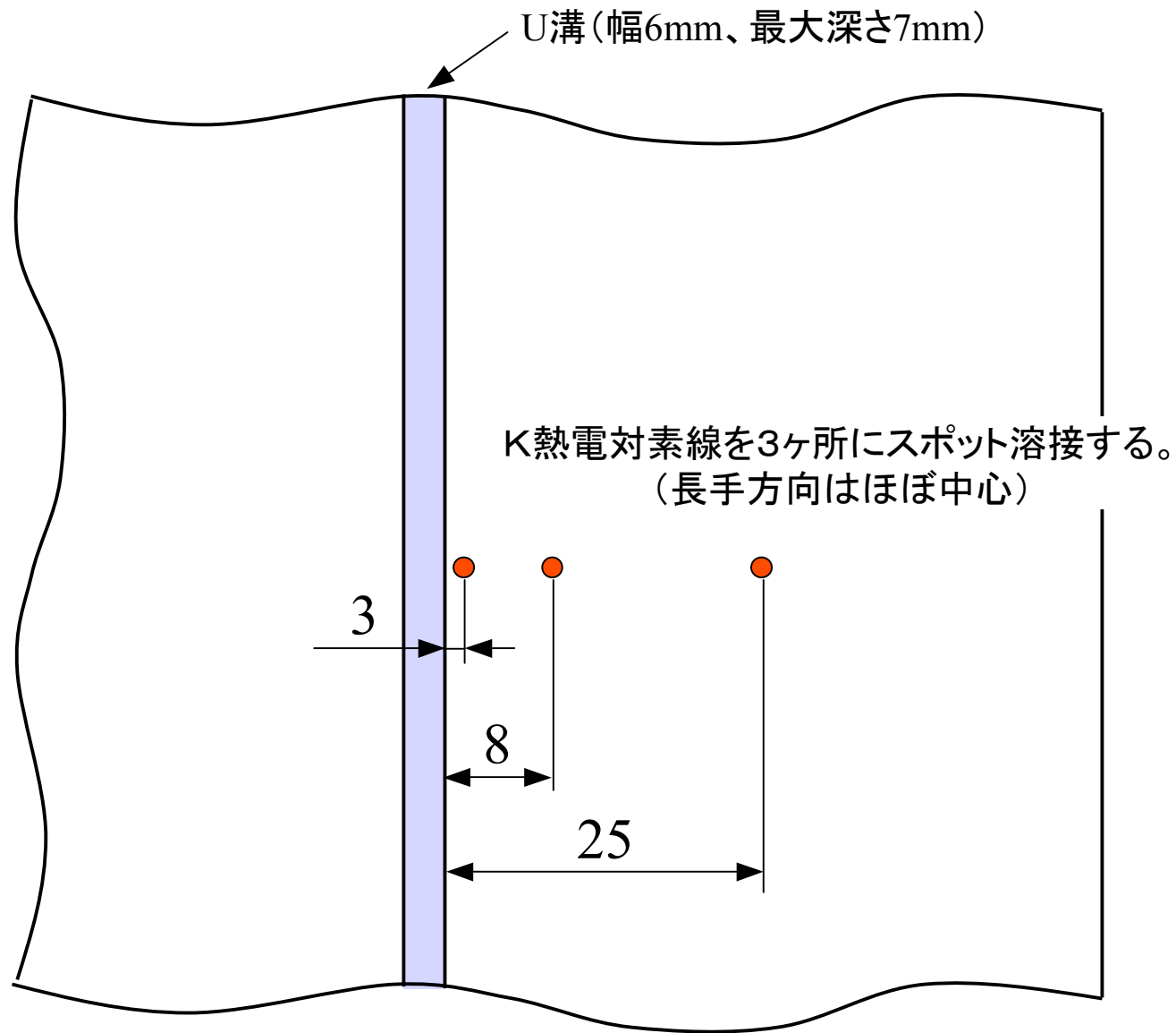
熱電対取り付け位置(SM570/SUS304)
